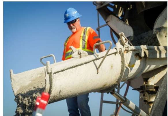
Coulage du béton de la fondation d'une tour sur le site canadien du pont
